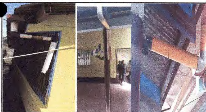
Foto 11: Sustrucción y reparación de bajadas de agua pluvial con tubo pvc
